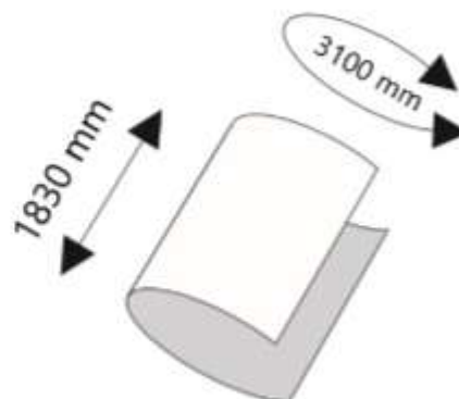
PREČNO KRIVLJENJE (1830 x 3100 mm)
